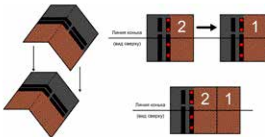
Рис. 26 Устройство рёбер скатов и коньков.
