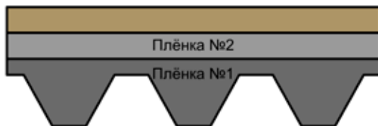
Рис. 13 Тыльная сторона гонта гибкой черепицы Döcke PIE.
