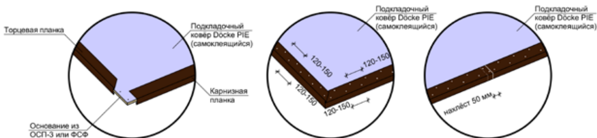
Рис. 8 Крепление металлических карнизных и торцевых планок.
