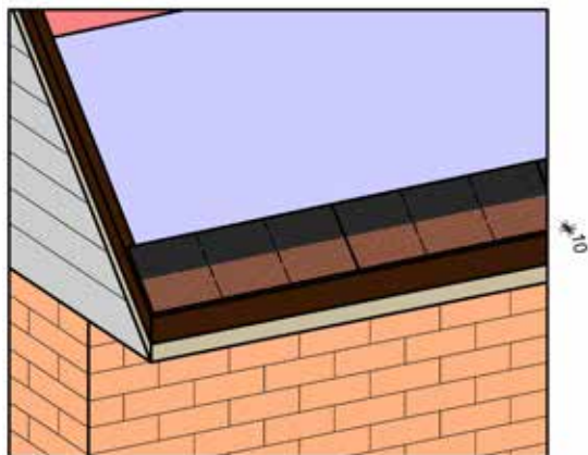
Рис. 11 Схема укладки карнизной черепицы на карниз.
