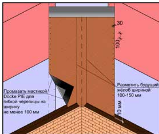
Рис. 9 Монтаж ендового ковра.
